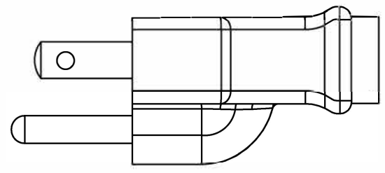
NEMA 5-20P (MSL-144)
